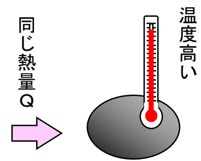
熱容量の小さな物体
