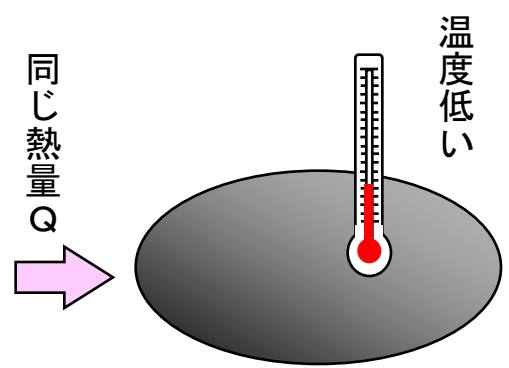
熱容量の大きな物体
