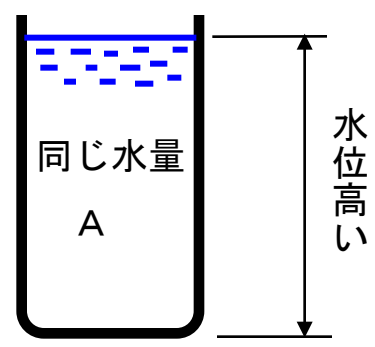
底の小さな容器
