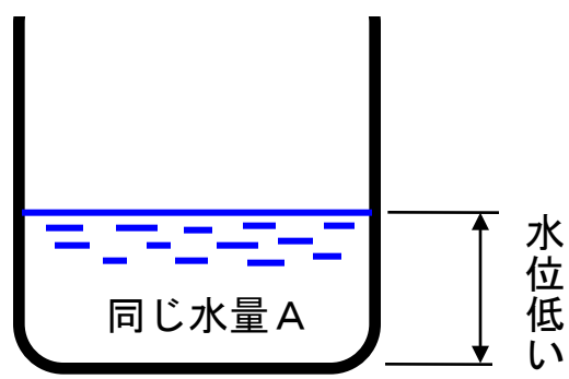
底の大きな容器
